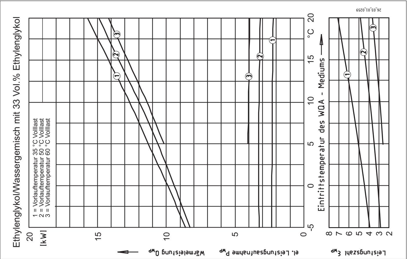
Leistungsdiagramm WPF 10
